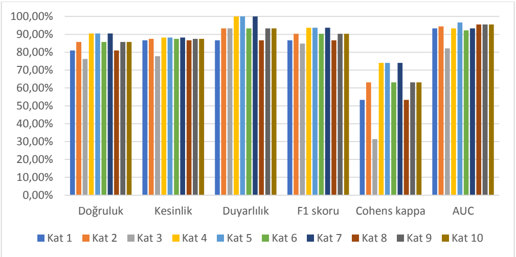
Grafik 1: 10-Katlı Çapraz Doğrulamaya Ait Sonuçlar
